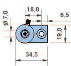
SUPORTE . SUPPORT E
