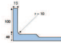
Alçado / Backplate
